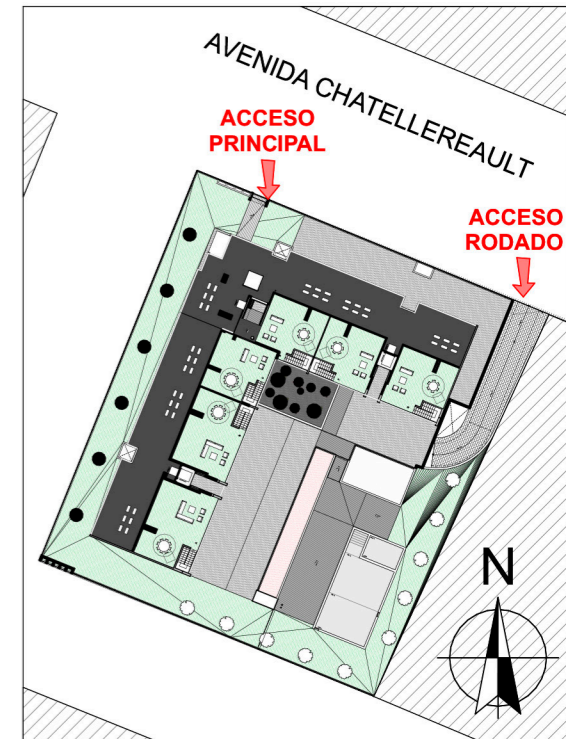
Planta Sótano -1
